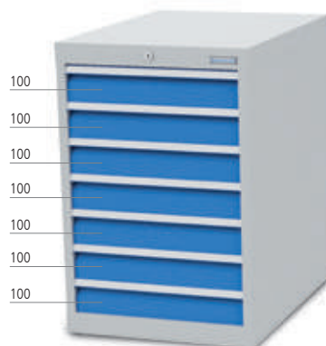
■ 7 x Schublade Art.-Nr. 580/0700V10A
