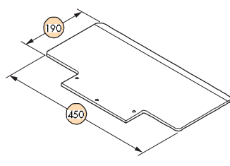
⑩ Art.-Nr. E/1543.930085 Schaufel DS-NG
