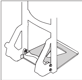
① Art.-Nr. E/1543.930103 Fixierte Schaufelbefestigung
